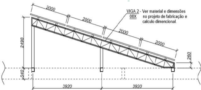
CORTE - ESTRUTURA PARA 4 PAINEIS
