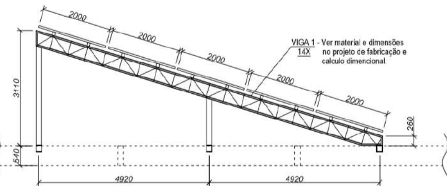
CORTE - ESTRUTURA PARA 5 PAINEIS
